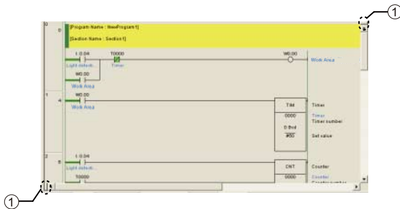
(1) Разделитель окна
