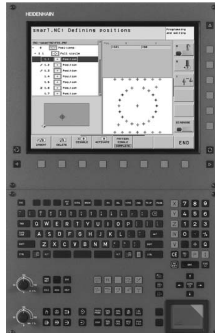
Плоский цветной монитор BF 150 с клавиатурой TE 530 B
