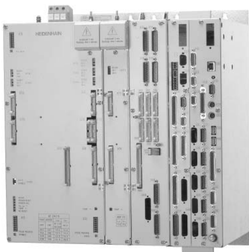
Основной компьютер и блок управления цифровыми приводами с компактным преобразователем и дополнительным силовым модулем
