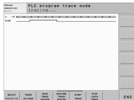
Логические диаграммы
